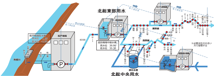
北総東部用水パイプラインシステム模式図
